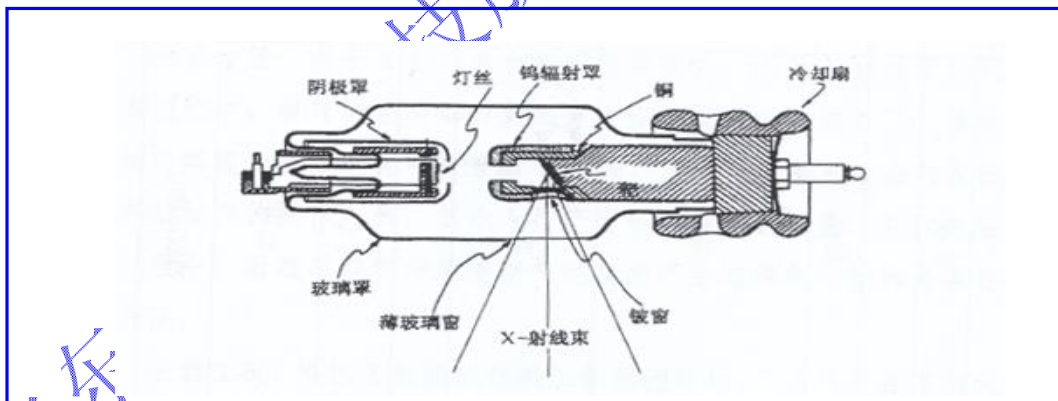
图 1 典型 X 射线管结构图
