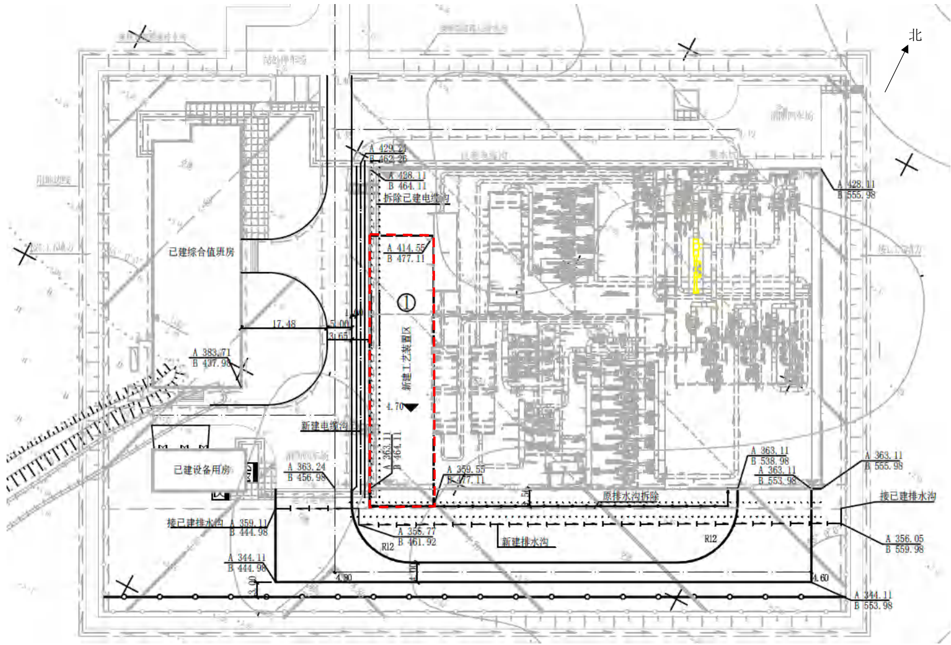
附图 11 厂区平面图(红色部分为本次新建工艺装置区)
